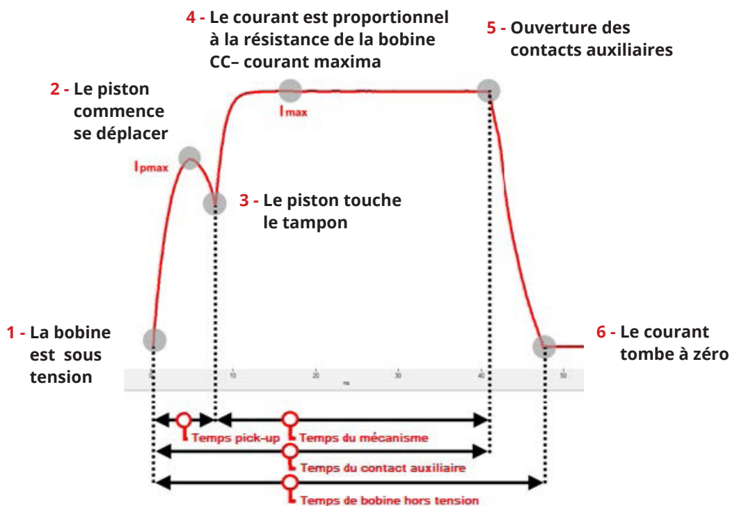
Figure 3. Points de courant de bobine spécifiques et paramètres de mesure
