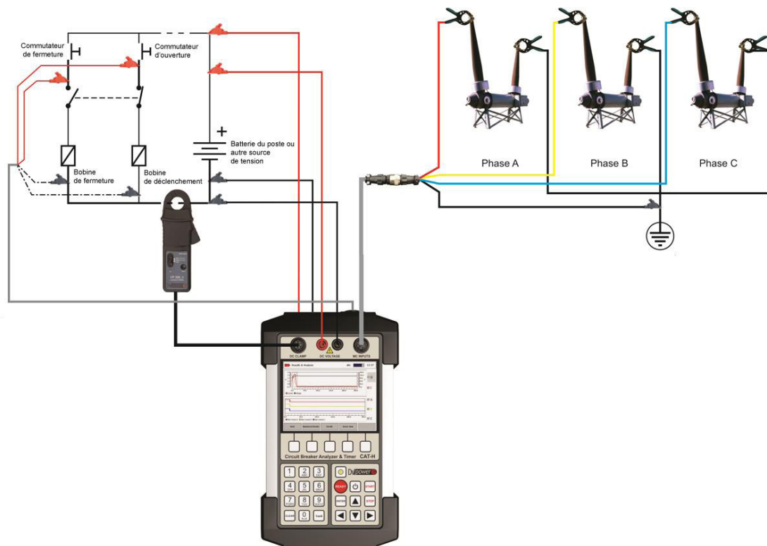
Figure 2. Branchement de CAT-H au disjoncteur à cuve mise à la terre avec 1 chambre de coupure par phase
