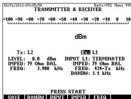
Trasmettitore e ricevitore in modo inseguimento.
