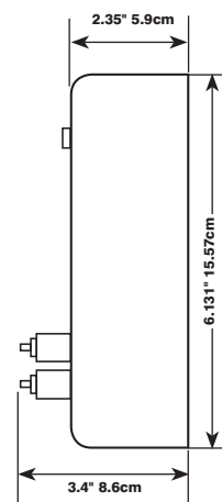
Vista Lateral del Nexus
