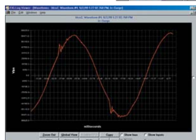
Transitorios de Sub-Ciclo
