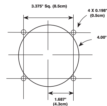
Pantalla Nexus P40N Patrón de Corte de Inserción
