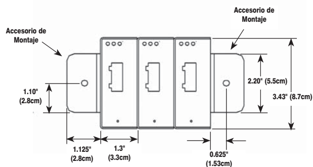
Módulos Nexus I/O Vista Frontal
