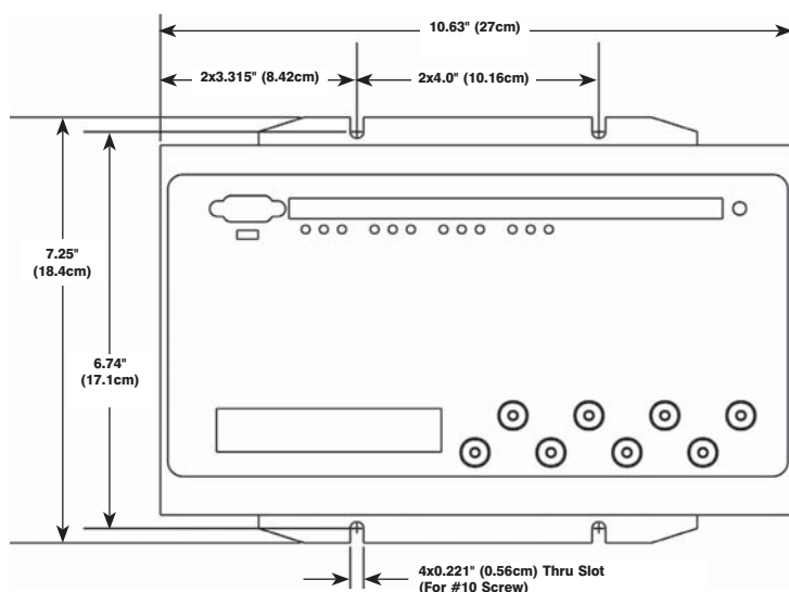
Vista Frontal del Nexus
