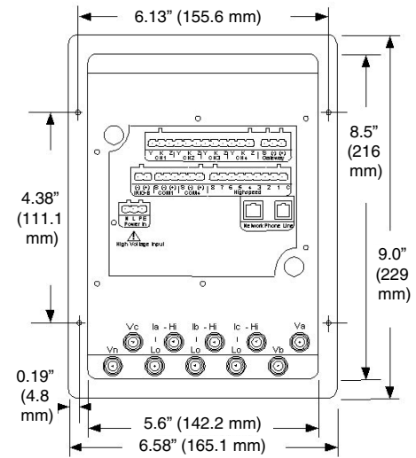
Nexus I/O Modules Corte Frontal
