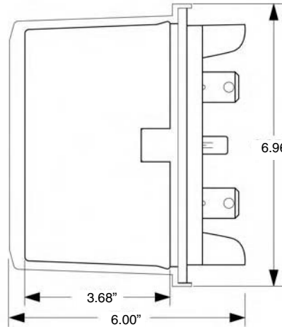
Nexus 1262/1272 Corte Lateral
