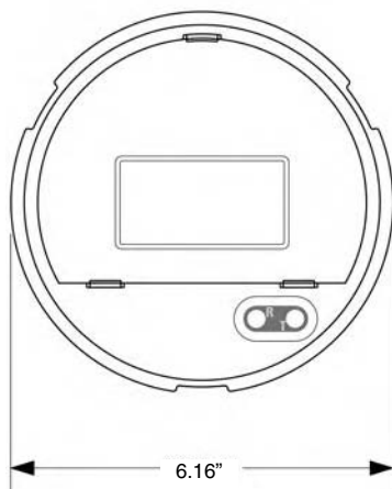
Nexus 1262/1272 Corte Frontal Cubierta Base A
