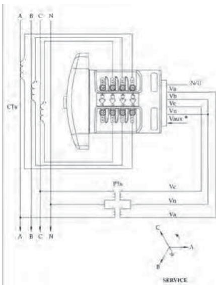
4 Hilos Estrella, 2,5 Elementos, 3 TCs y 2 TPs
