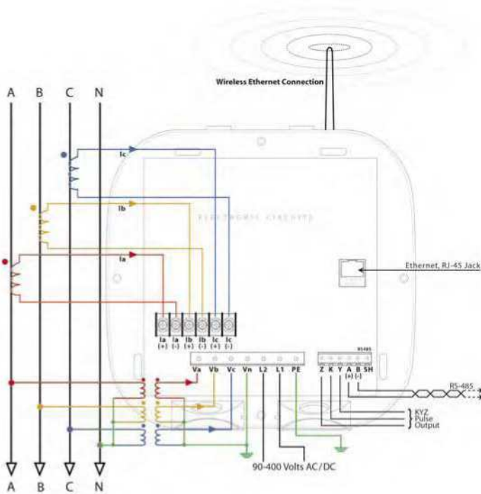
4 Hilos, 3 Fases " Y " con PTS
