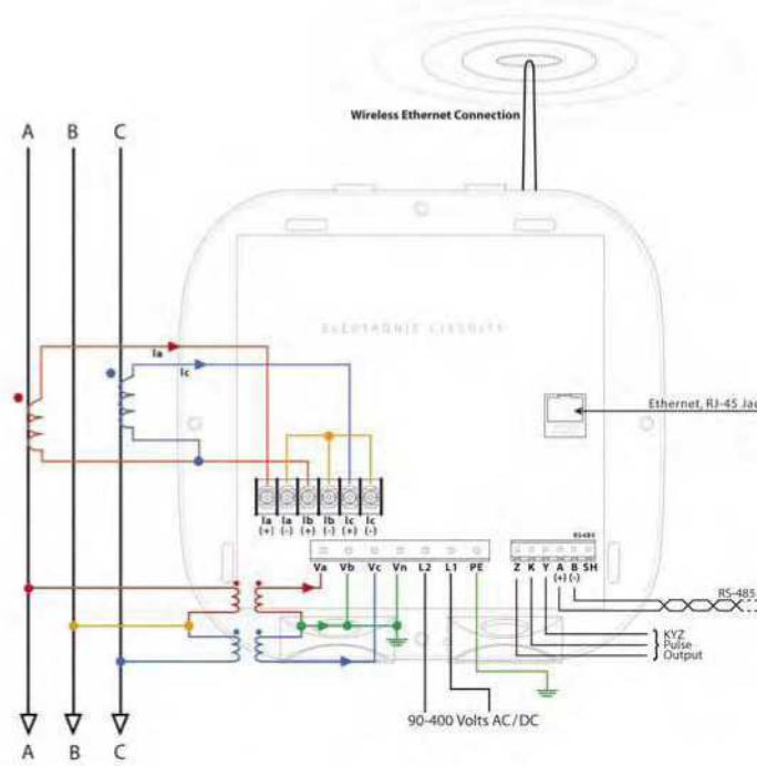
3 Hilos, 3 Fases Delta con PTS
