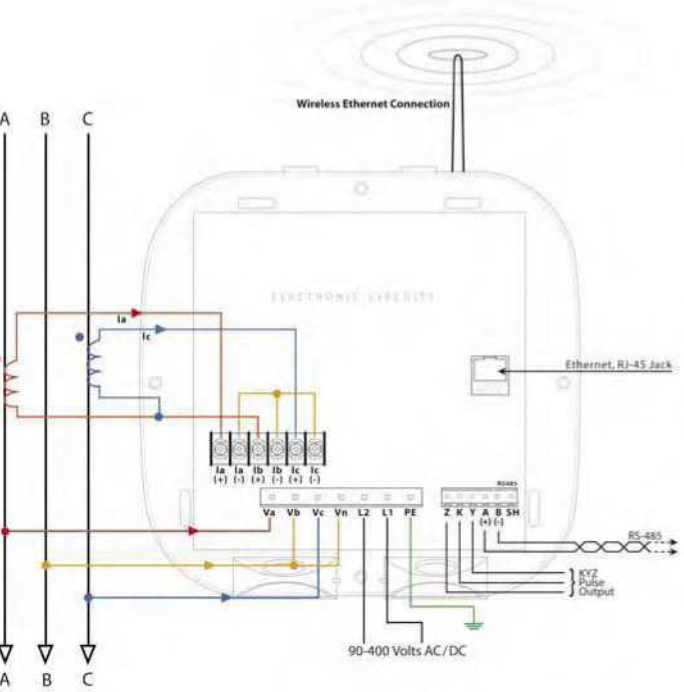
3 Hilos, 3 Fases Delta Directo
