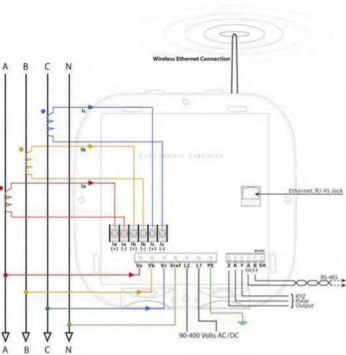
4 Hilos, 3 Fases " Y "
