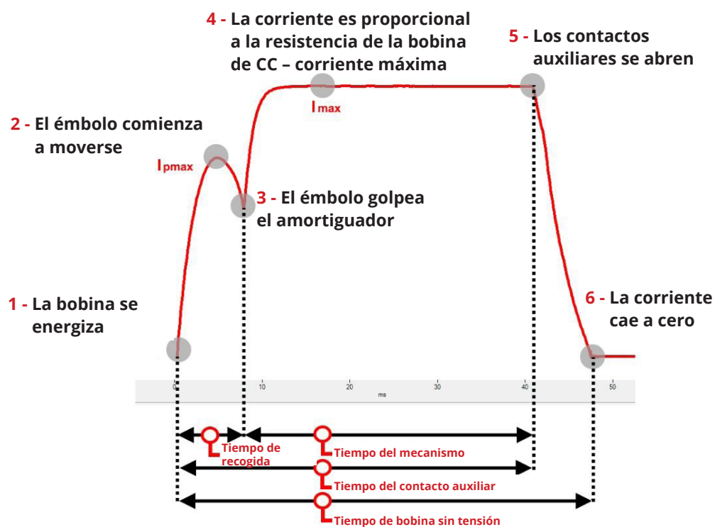
Figura 3. Puntos específicos de la corriente de bobina y parámetros de medición
